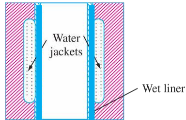
b) wet liner
